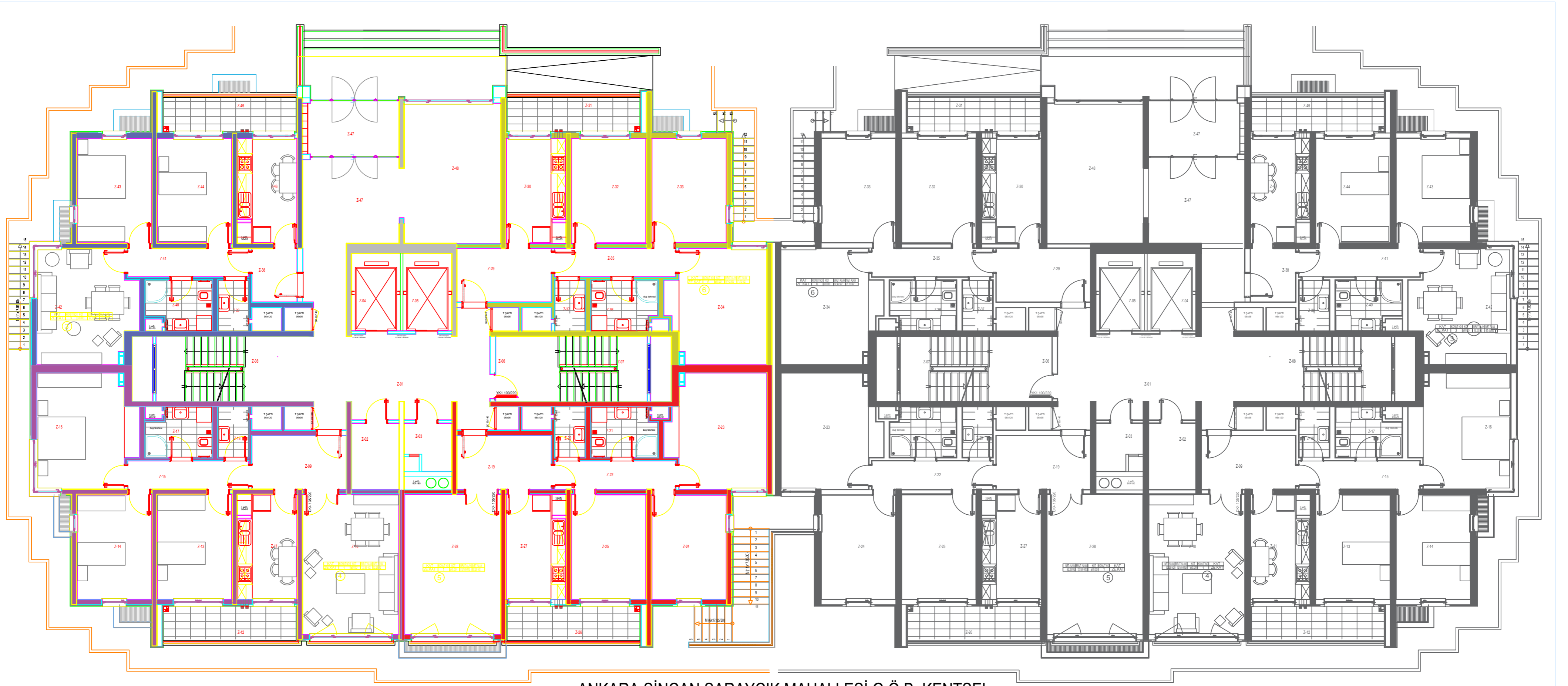
ANKARA SINCAN SARAYCIK MAHALLESİ G.Ö.B. KENTSEL DÖNÜŞÜM PROJESİ SC3 TİP BLOK ZEMİN KAT PLANI
